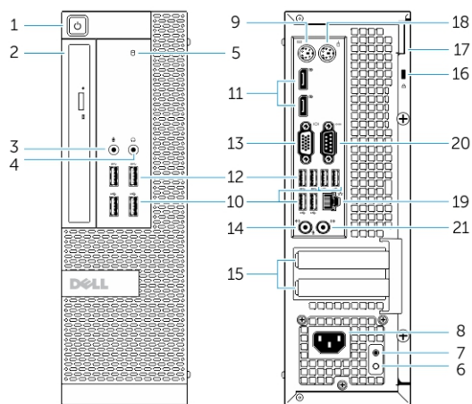
Skica 1. Pogled s sprednje in zadnje strani
