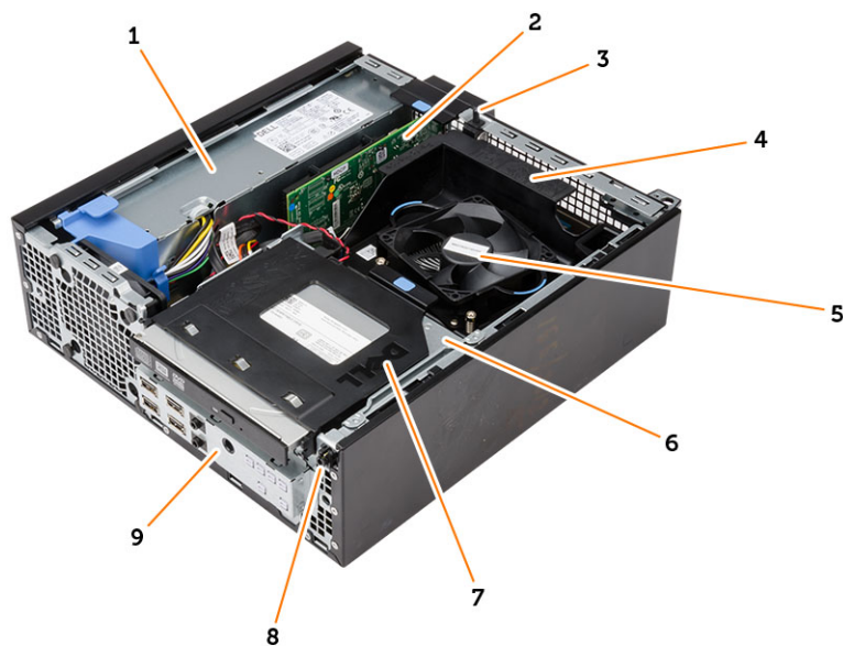
Skica 2. Vpogled v notranjost vašega računalnika
